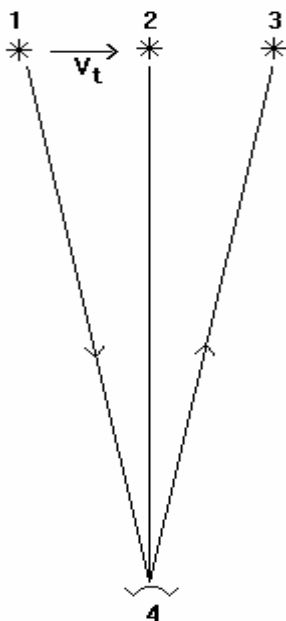
Рис.1 "Прошное" (1), "истинное" (2) и "будущее" (3) положения астрономического объекта. Порция света, излученная объектом, находящимся в положении (1), через много лет доходит до наблюдателя (4). За это время объект, двигающийся перпендикулярно направлению к наблюдателю со скоростью V_t , перемещается в положение (2). Если бы в момент регистрации порция света была бы излучена из места наблюдения, она встретила бы с объектом в точке (3).
