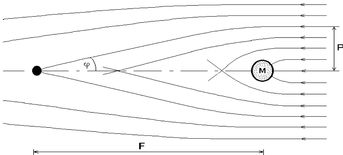
Рис.2. Фокусировка неподвижным гравитирующим объектом. Проходящий со скоростью V на расстоянии от центра объекта p = (2GMF)^{1/2} / V поток агента "схлопывается" в точке наблюдения. Наблюдатель воспринимает приходящий поток как кольцо с угловым радиусом \phi \approx p/F .
