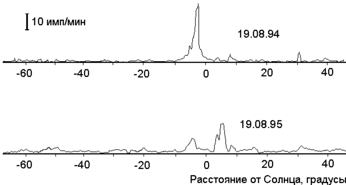
Рис.5. Всплески сигнала во время сближения центра Солнца со звездой \nu Льва (минимальное расстояние 5 угловых минут). Телескоп: стальное параболическое зеркало с фокусным расстоянием 10 см, детектор - счетчик Гейгера диаметром 2 мм и длиной 6 мм [8].
