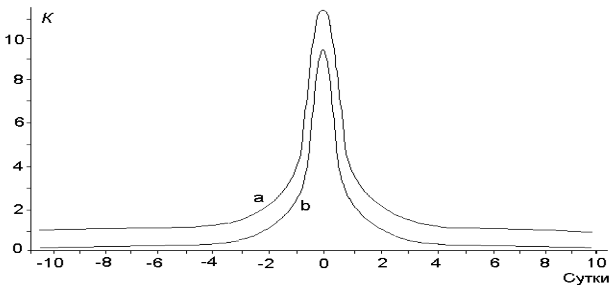
Рис.4. Расчетное изменение плотности потока проходящих вблизи Солнца мононаправленных частиц, имеющих скорость 500 \text{ км/с} , при угловом сближении направления потока и направления на центр Солнца (минимальное расстояние - 12 угловых минут) [13]. По горизонтальной оси - время от момента наиболее тесного сближения; a - первичный "источник", b - возникающий и исчезающий "источник".
