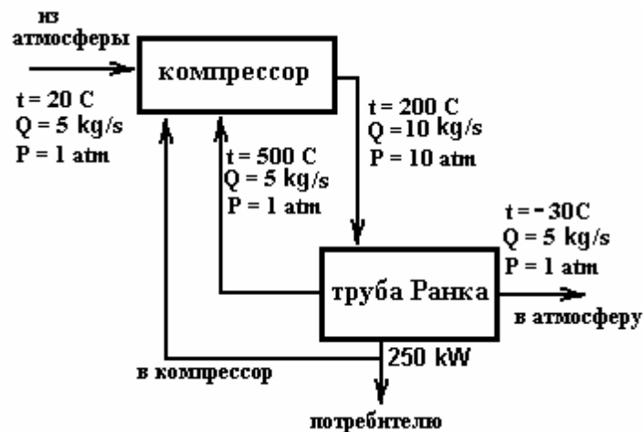
Рис 3. Энергетическая установка
