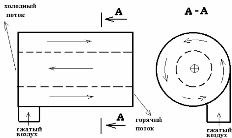
Рис 2. Вихревая труба Ранка (схема)
