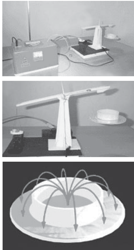
Рис. 3. Конденсатор Фролова по версии Жана Нода (Jean L. Naudin)
