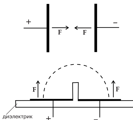
Рис. 2. Т-образный конденсатор Фролова
