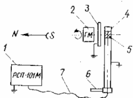
Рис. 15. Схема эксперимента из [50].
